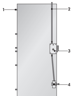
Vulcano REI 60 a cilindro
