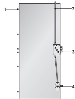
Vulcano REI 90
