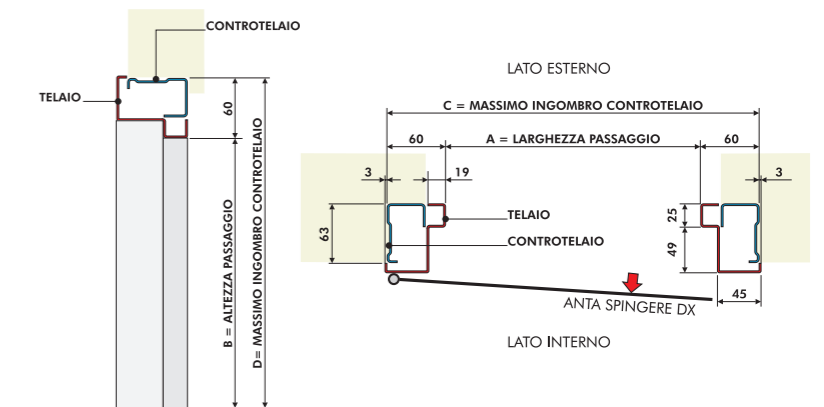
MISURE STANDARD PER IL TELAIO E CONTROTELAIO
