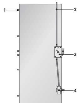
Vulcano REI 60
