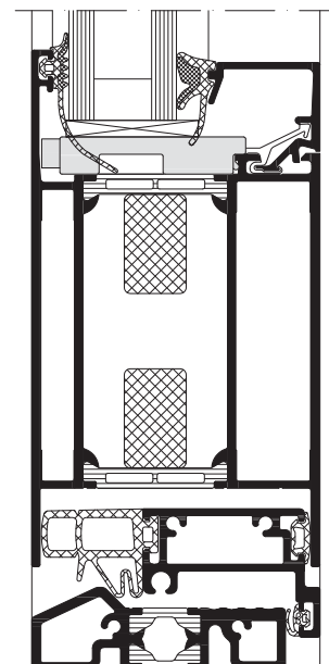
Schüco Tür ADS 75.SI, Maßstab 1:2 Schüco Door ADS 75.SI, Scale 1:2
